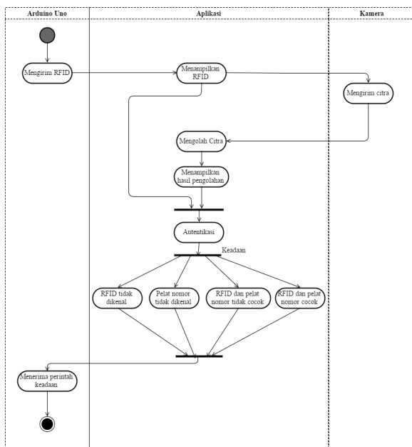
Gambar 8. Diagram aktivitas autentikasi
