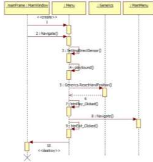
Gambar 4. Sequence Diagram untuk Use Case Mulai Aplikasi
