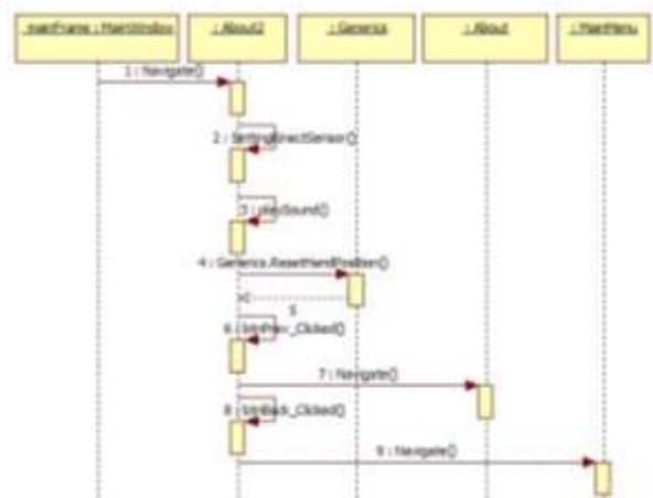
Gambar 11. Sequence Diagram kredit suara latar untuk Use Case Kredit Permainan
