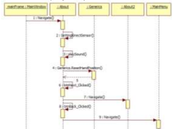
Gambar 10. Sequence Diagram pengembang permainan untuk Use Case Kredit Permainan
