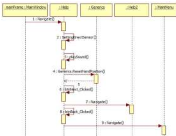
Gambar 8. Sequence Diagram perkenalan karakter untuk Use Case Cara Bermain
