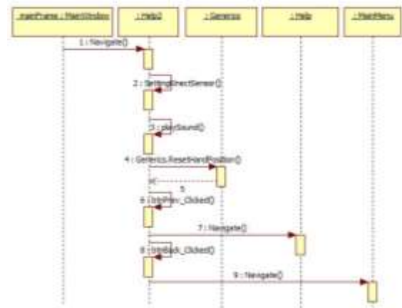
Gambar 9. Sequence Diagram petunjuk permainan untuk Use Case Cara Bermain
