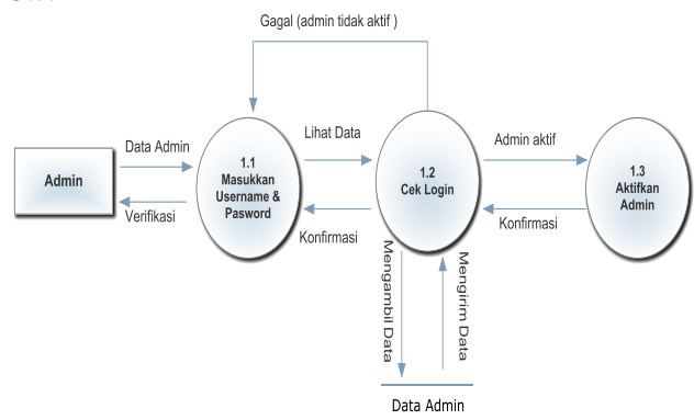
Gambar 3.7 DFD proses pertama
