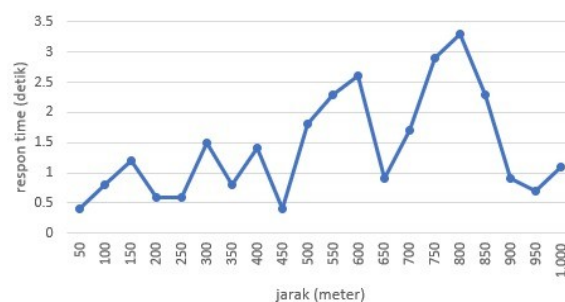
Gambar 7. Waktu respons sistem terhadap jarak pengontrol berbasis aplikasi
