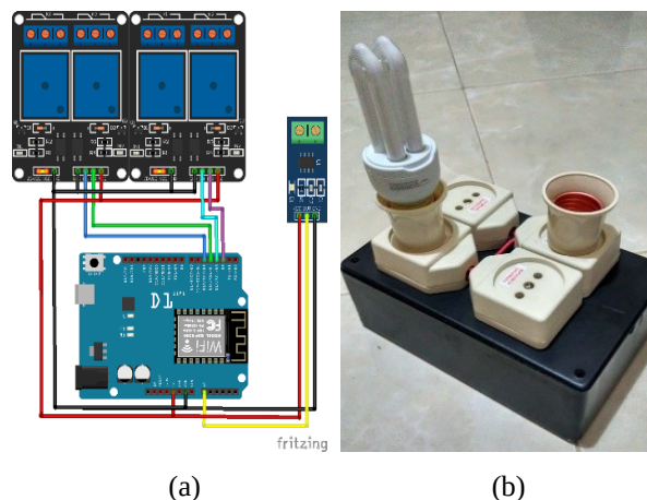
Gambar 4. Skematik rangkaian dan perangkat saklar
