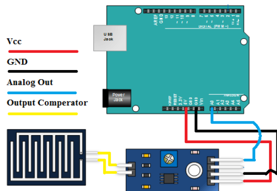
Gambar 10. Pengawatan sensor rintik hujan
