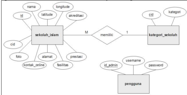
Gambar 7 Desain ERD SIG sekolah Islam
