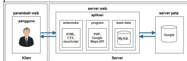
Gambar 6 Arsitektur aplikasi SIG sekolah Islam
