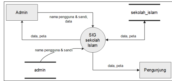
Gambar 9 Diagram Konteks SIG sekolah Islam
