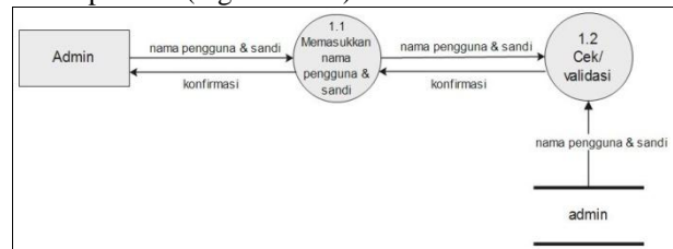
Gambar 11 Diagram Aliran Data level 1 proses 1 SIG sekolah Islam
