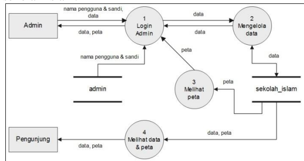
Gambar 10 Diagram Aliran Data Level 0 SIG sekolah Islam
