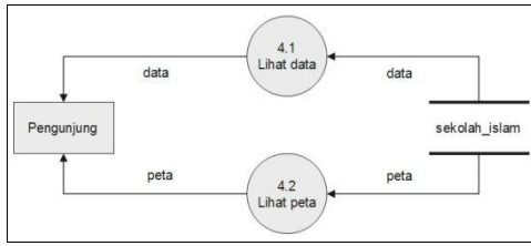
Gambar 13 Diagram Aliran Data level 1 proses 4 SIG sekolah Islam
