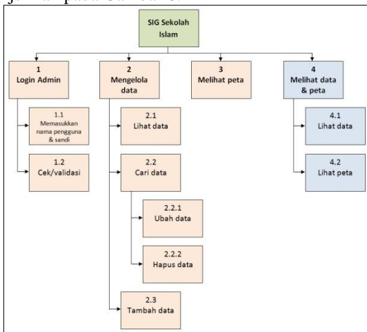
Gambar 8 Dekomposisi diagram SIG sekolah Islam
